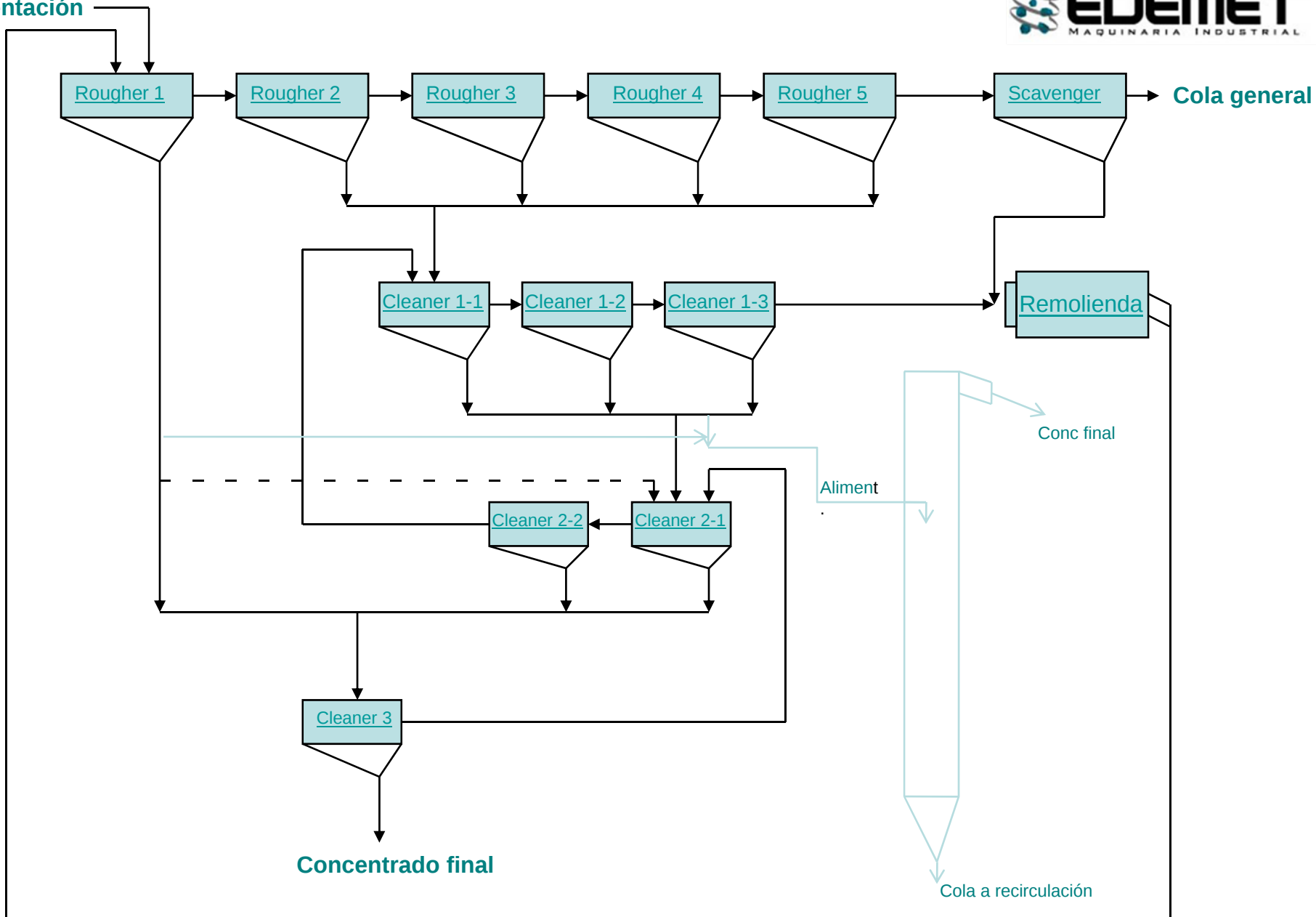
Figura: Flowsheet tentativo para flotación con MPPFE de EDEMET
